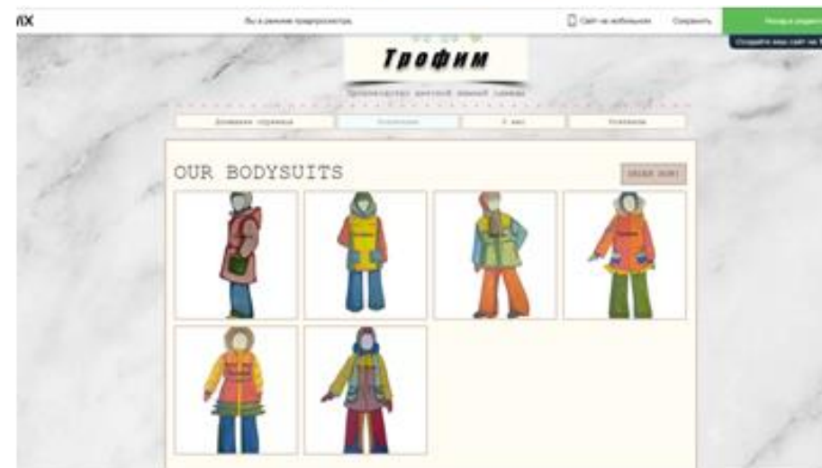
Рисунок 10 – Вкладка «коллекции»
