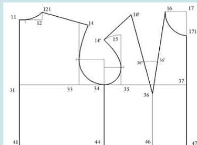
Рис.1 – Развертка верхней опорной поверхности
