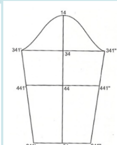
Рис.2 – Развертка поверхности рукава
