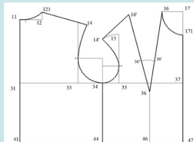
Рис.1 – Развертка верхней опорной поверхности
