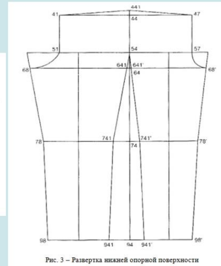
Рис.3 – Развертка нижней опорной поверхности
