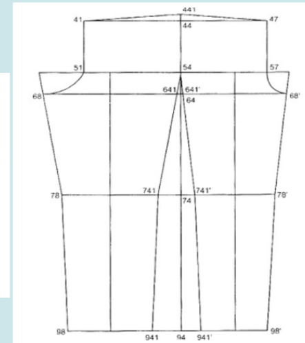
Рис.3 – Развертка нижней опорной поверхности
