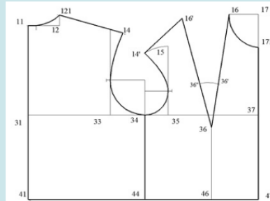
Рис.1 – Развертка верхней опорной поверхности
