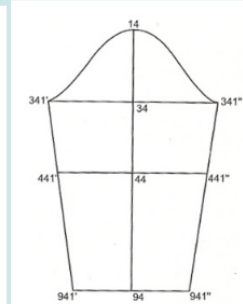
Рис.2 – Развертка поверхности руки
