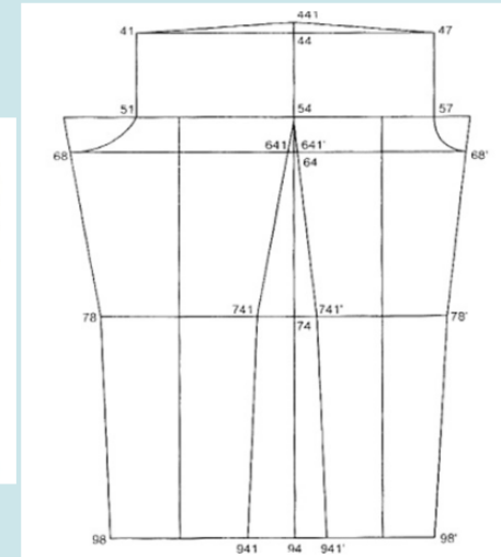
Рис.3 – Развертка нижней опорной поверхности
