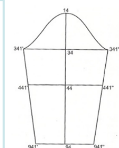
Рис.2 – Развертка поверхности руки
