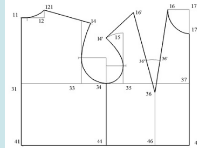
Рис.1 – Развертка верхней опорной поверхности
